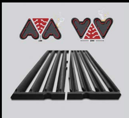
Těžké oboustranné rošty z litiny
